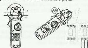
Obrázok 2 - Meranie prúdu
